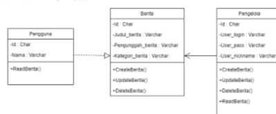
Gambar 6. Class Diagram di Laman Berita
